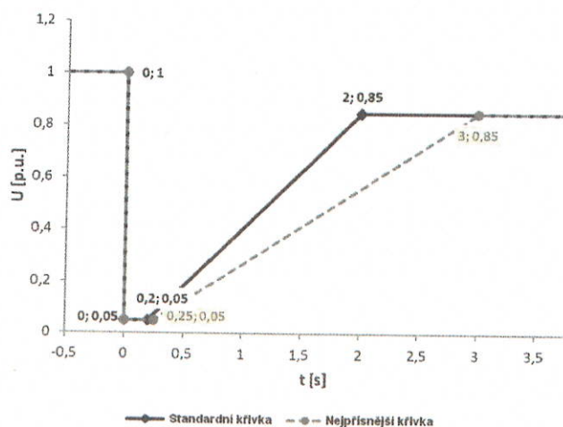
Obr. 2 Schopnost překlenutí poruchy pro výrobny se střídačem na výstupu
