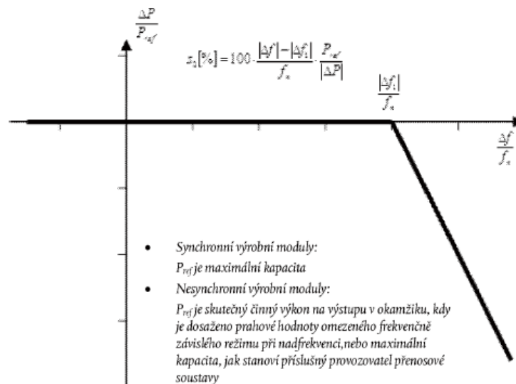
Obr. 1 Diagram LFSM-O
