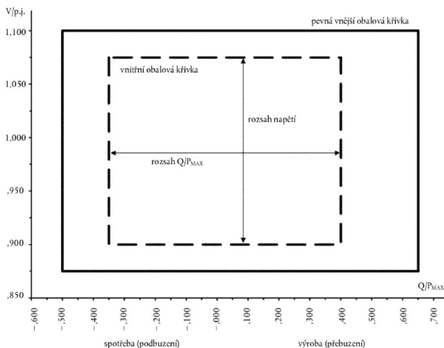
Profil U-Q/P max nesyndronního výrobního modulu.
