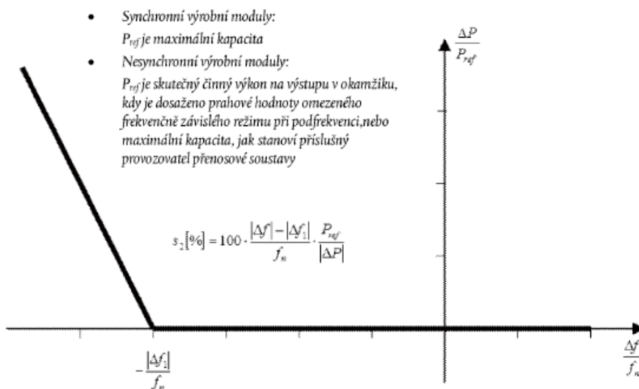
Obr. 6 Diagram LFSM-U
