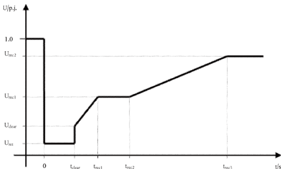
Profil schopnosti výrobního modulu překlenout poruchu.
